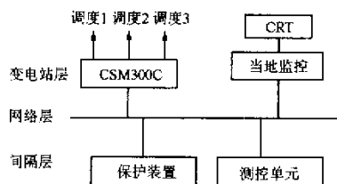
图 1 CSC2000 系统结构图
