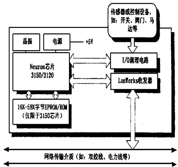
图2 基于 Neuron 芯片智能节点结构图
